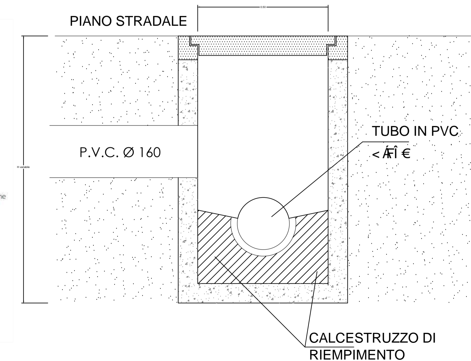
Particolare pozzetto acque nere
