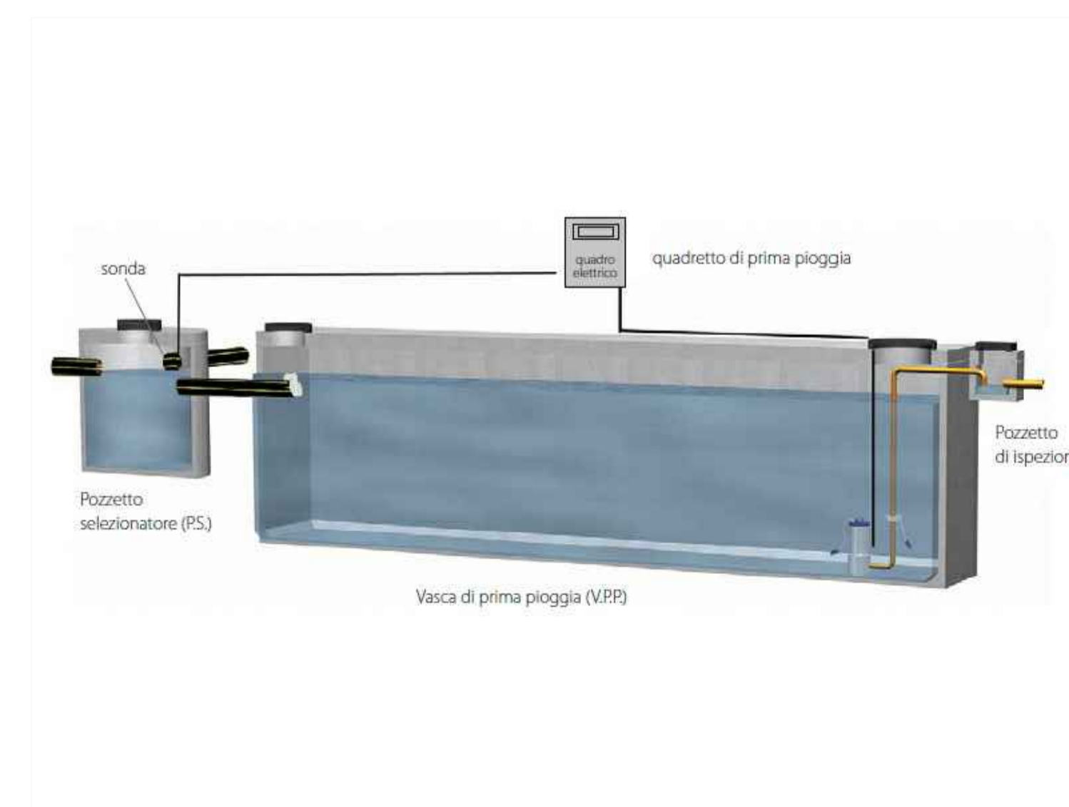
Particolare vasche di accumulo
